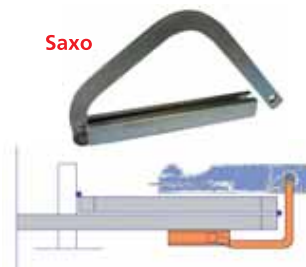
Desbloqueo externo. Conjunto de herrajes que permiten el desbloquear el operador desde el exterior (necesita maneta).
